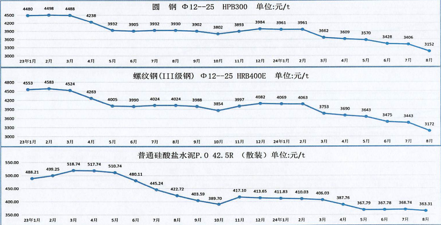
2024 年 8 月广州地区建设工程部分常用材料税前综合价格走势图
